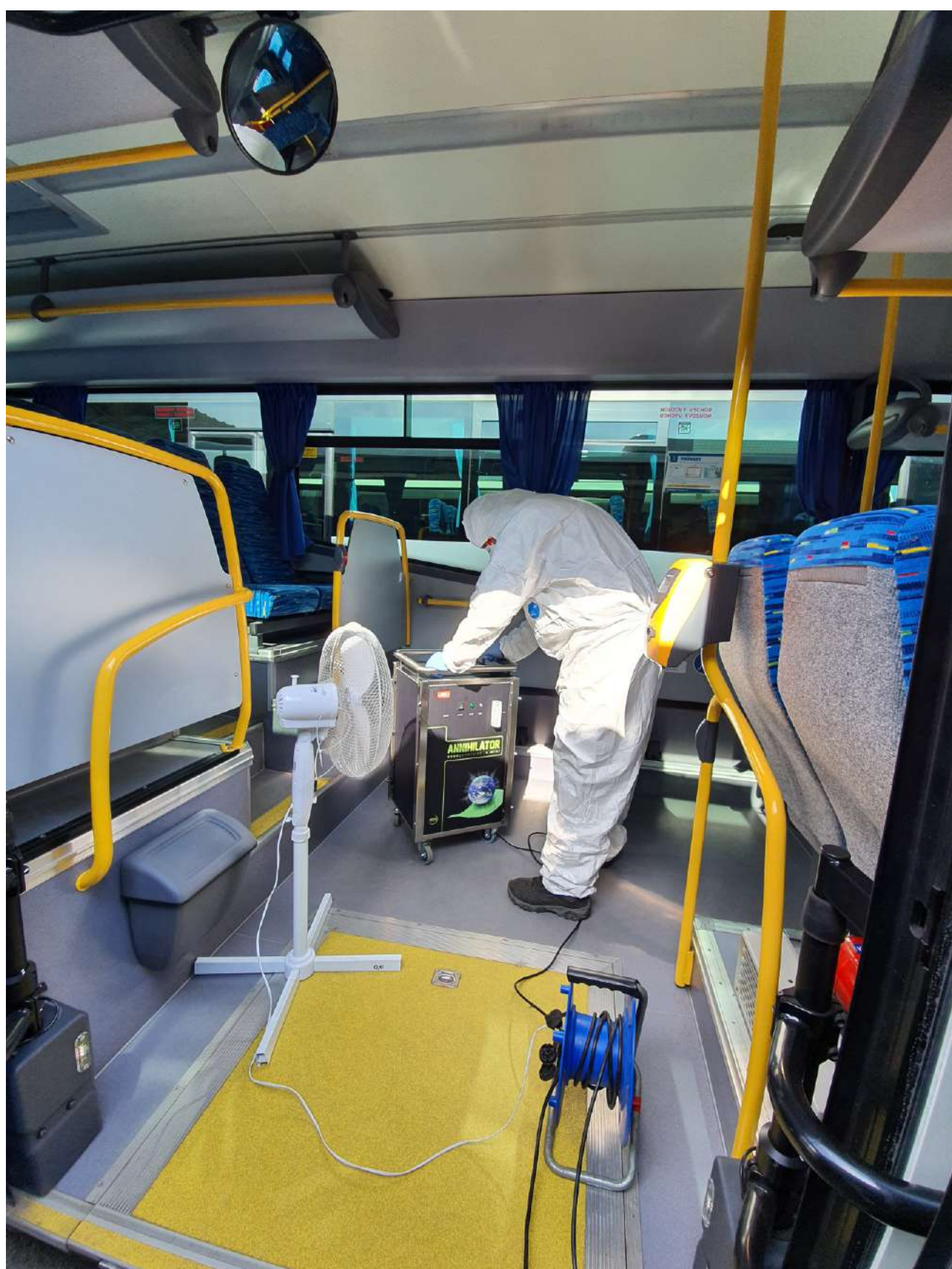
rychlejší rozptýlení ozonu po prostoru podporujeme ventilátorem
